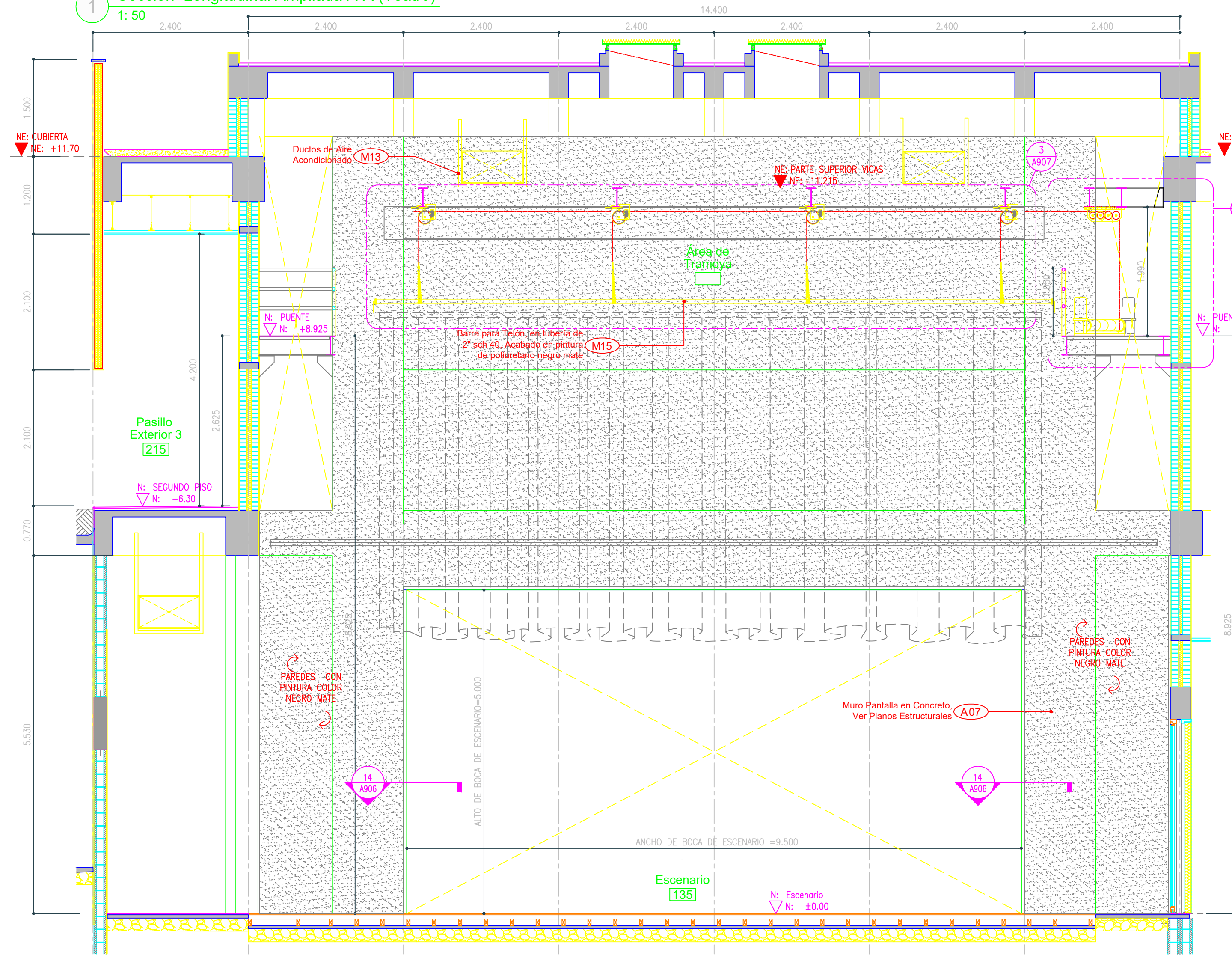
1 Sección Longitudinal Ampliada A-A (Teatro) 1:50
