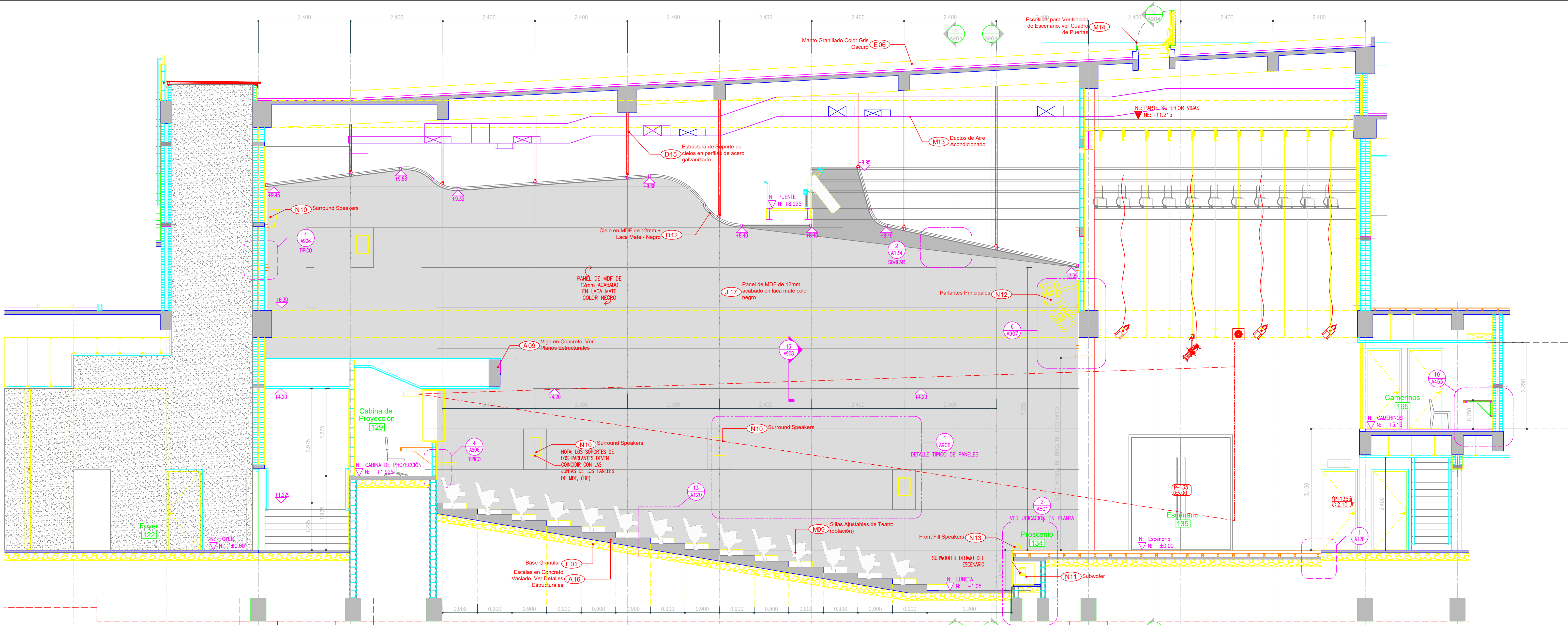
1 Sección Longitudinal Ampliada A-A (Teatro) 1:50
