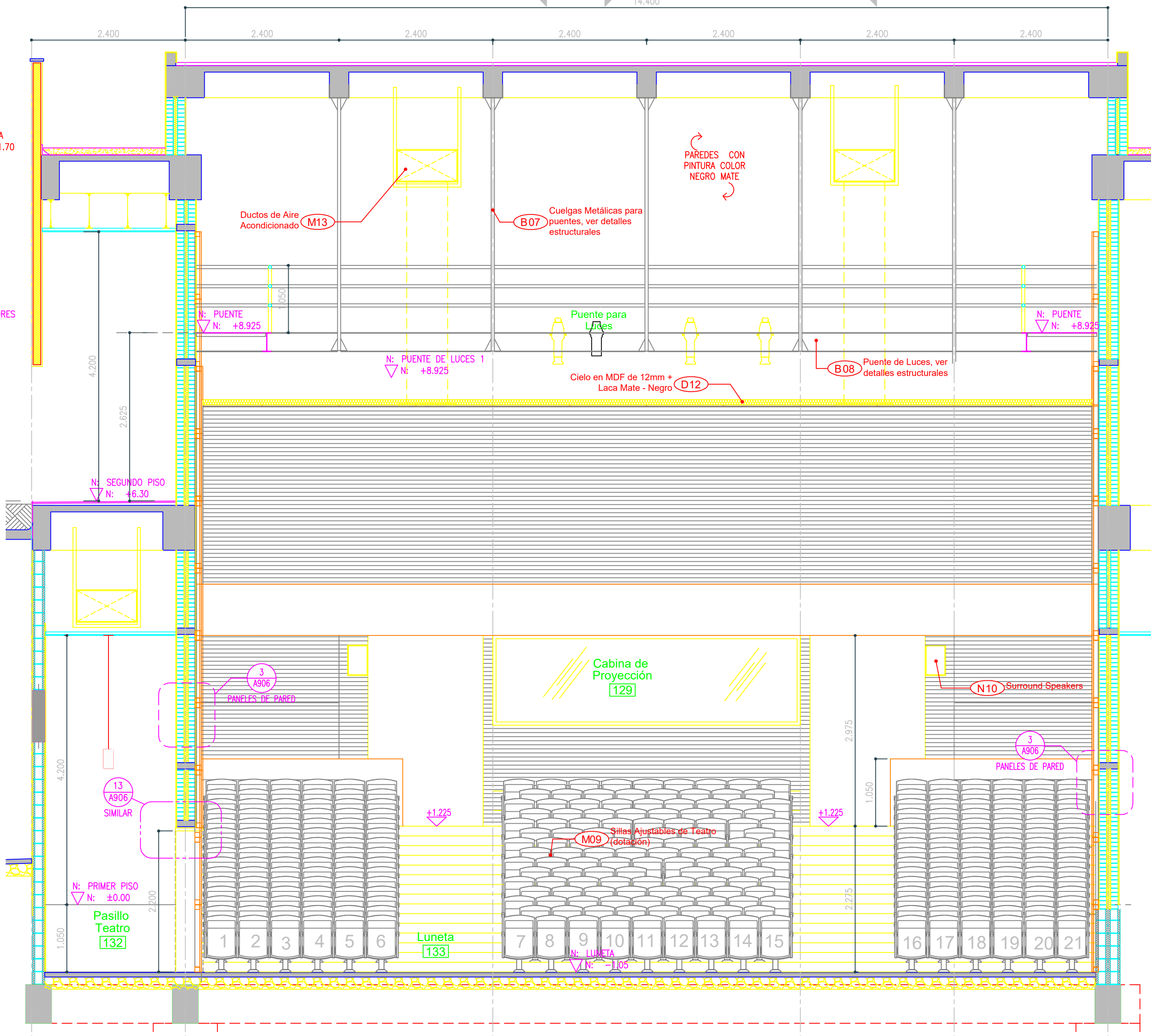
3 Sección Transversal Ampliada Q-Q (Teatro) 1:50
