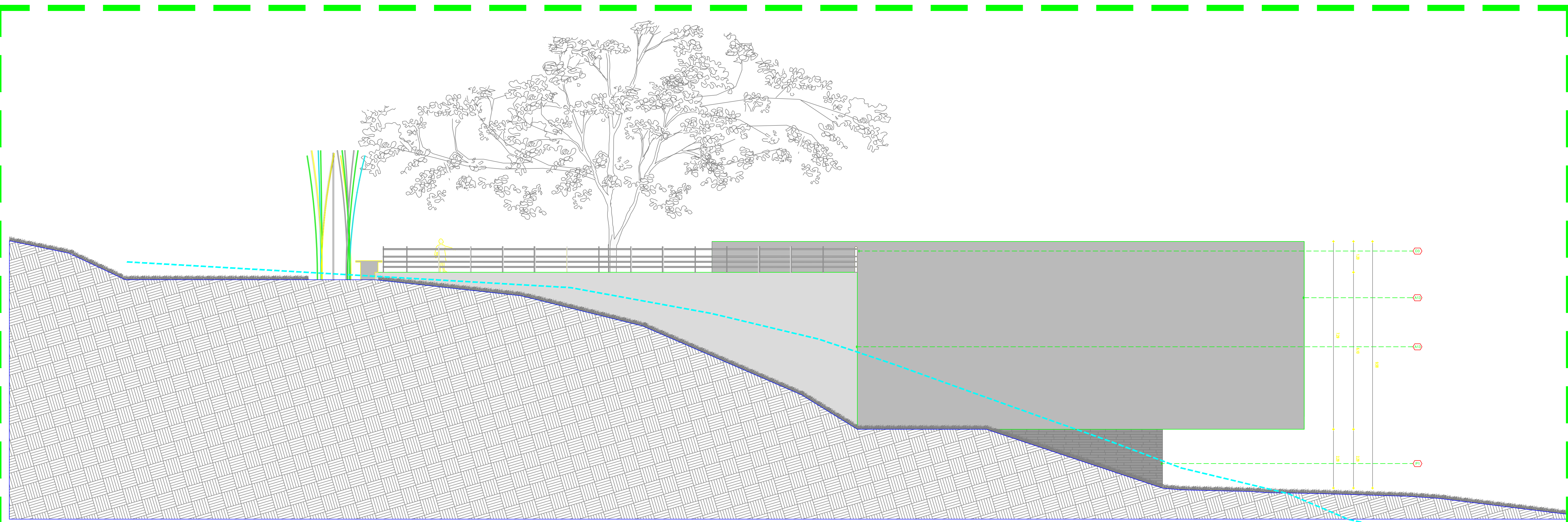
FACHADA 8 ESCALA 1:75
