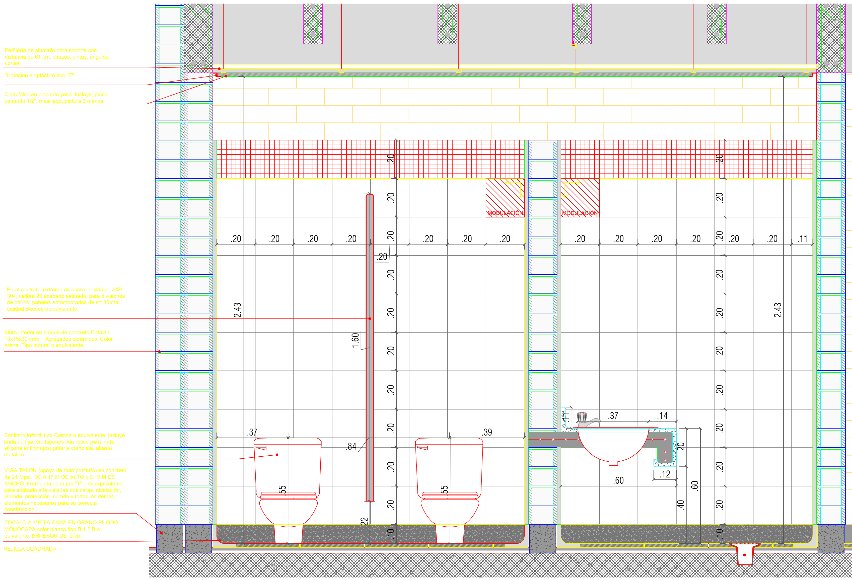
Baños Infantiles - Seccion D-D ESC 1:20
