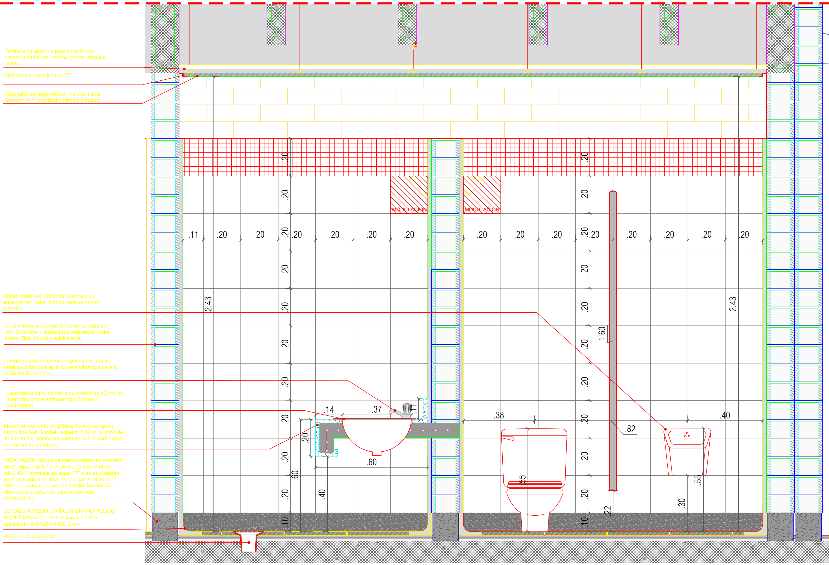
Baños Infantiles - Seccion C-C ESC 1:20
