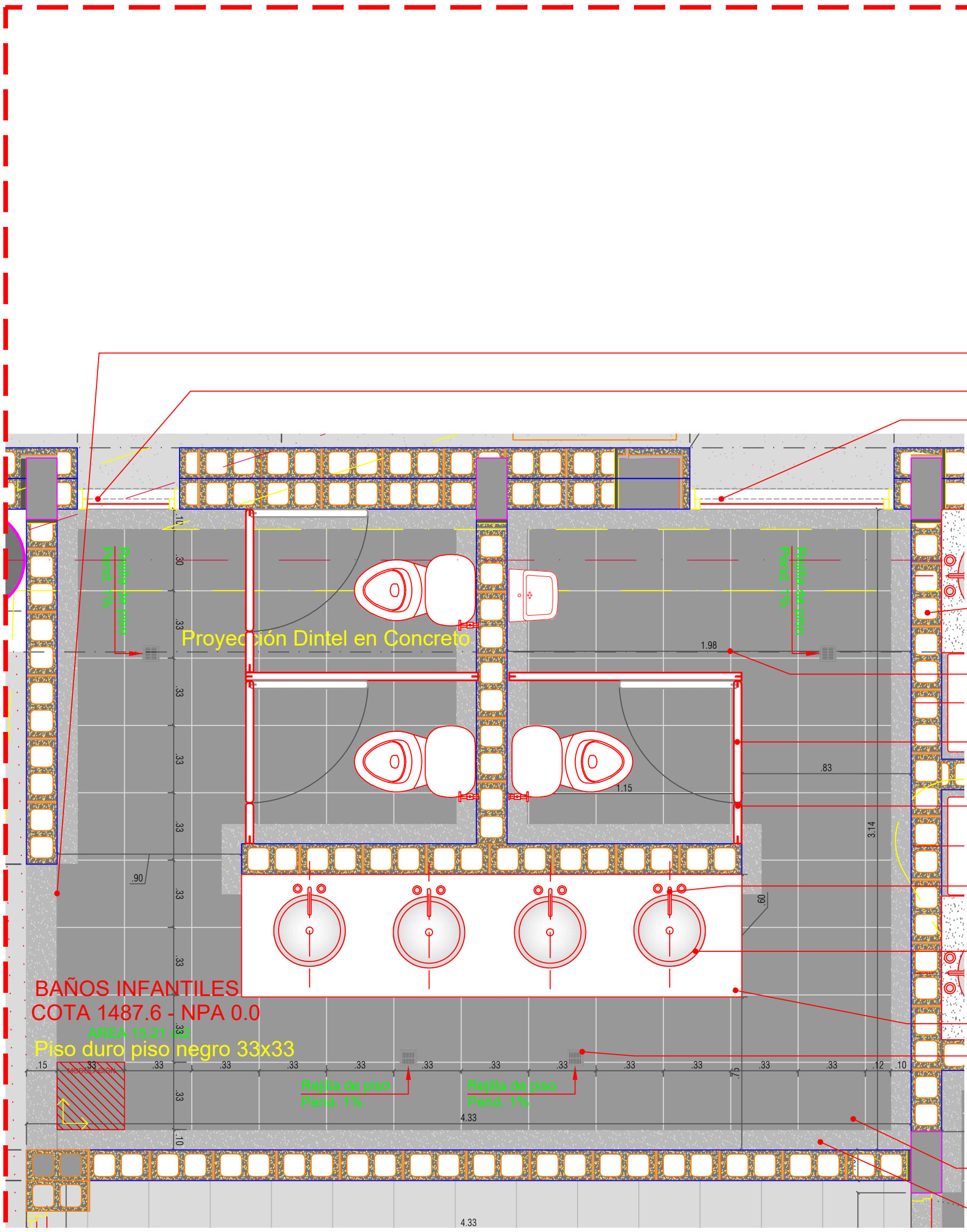
Baños Infantiles - Planta ESC 1:20
