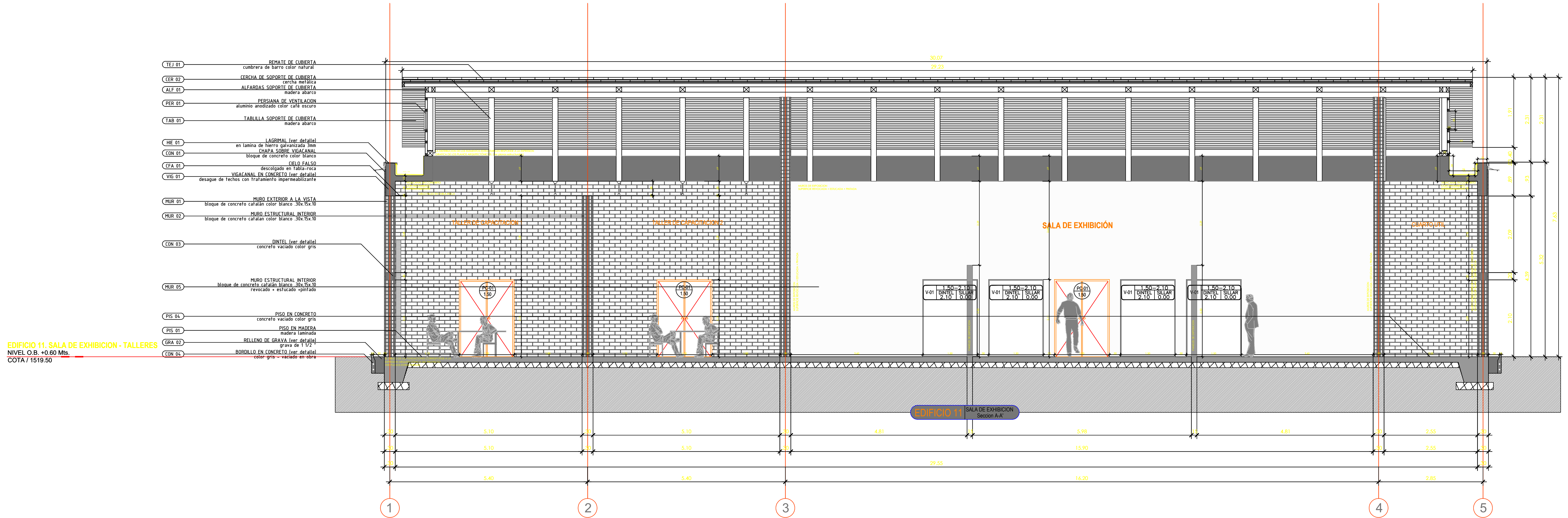
SECCION A - A' ESC. 1:50
