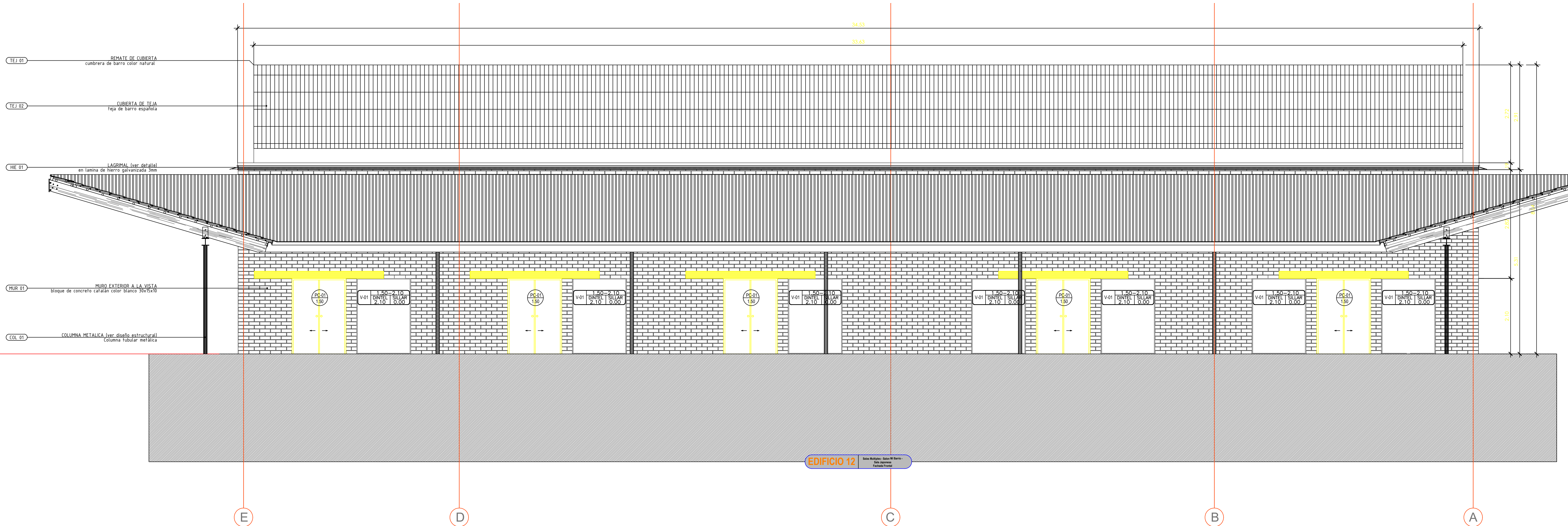
FACHADA FRONTAL ESC. 1:50
