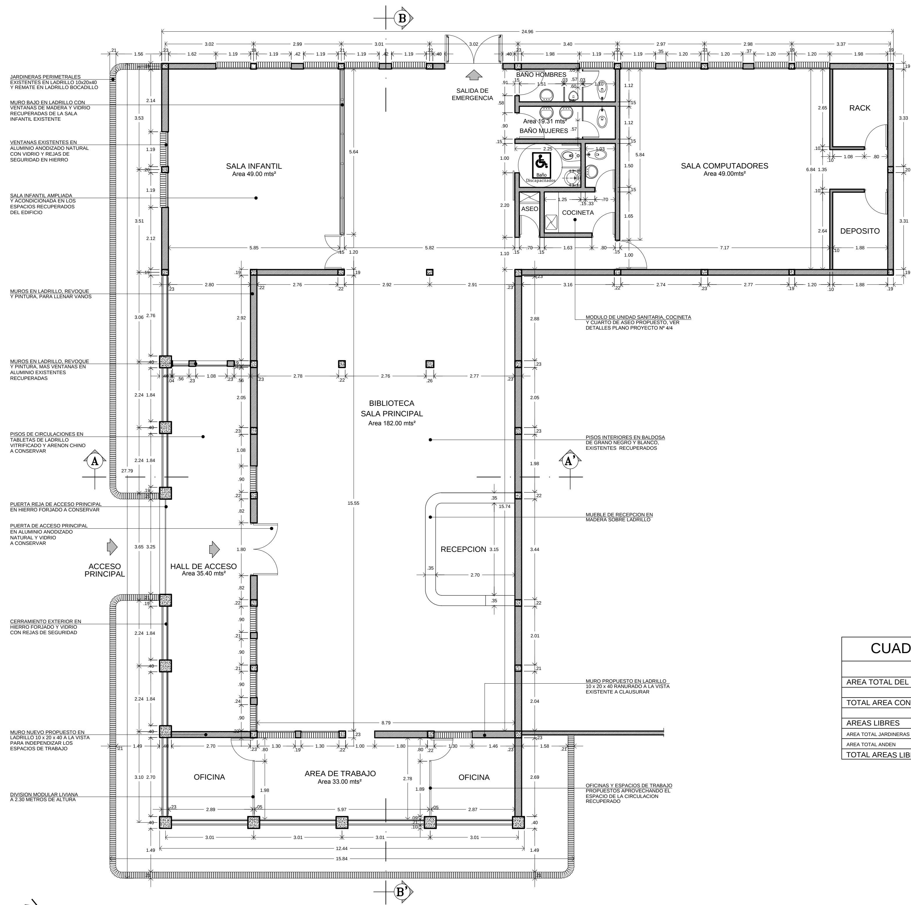
BIBLIOTECA EXISTENTE PROPUESTA DE READECUACION PLANTA GENERAL
