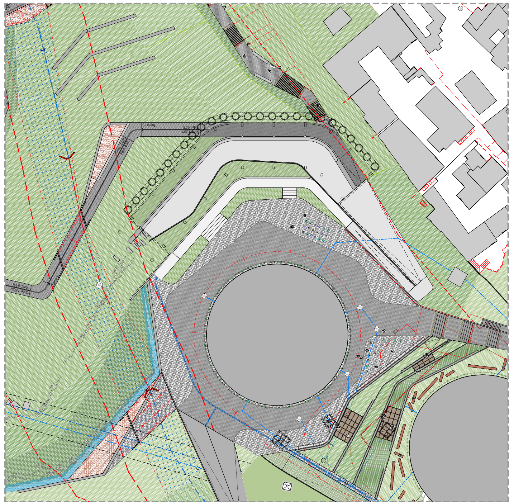
PLANTA DE CONTEXTO URBANO ESC 1:500
