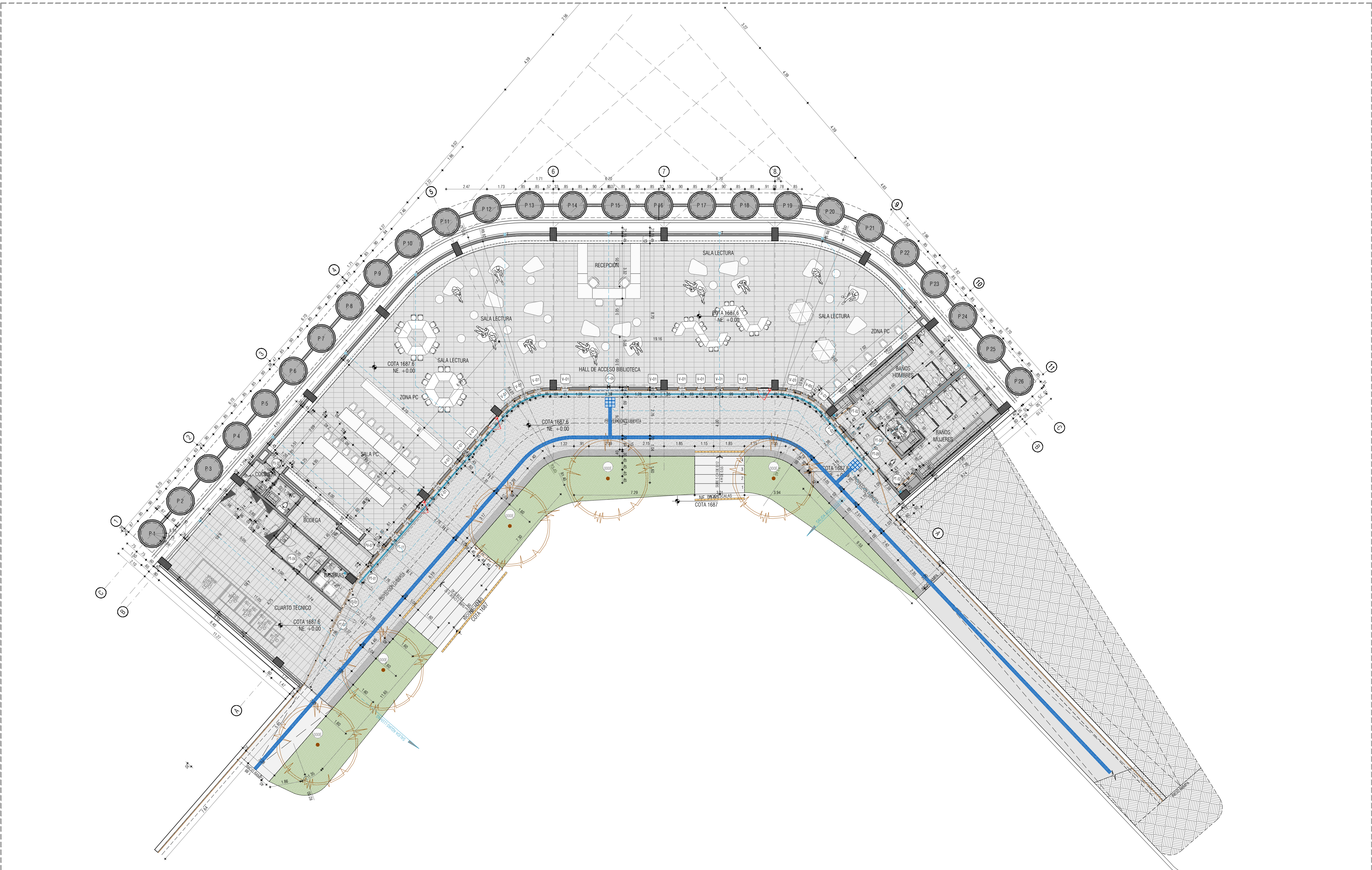
UPO-CU-001/ Planta piso 1 (programa) ESC 1:125
