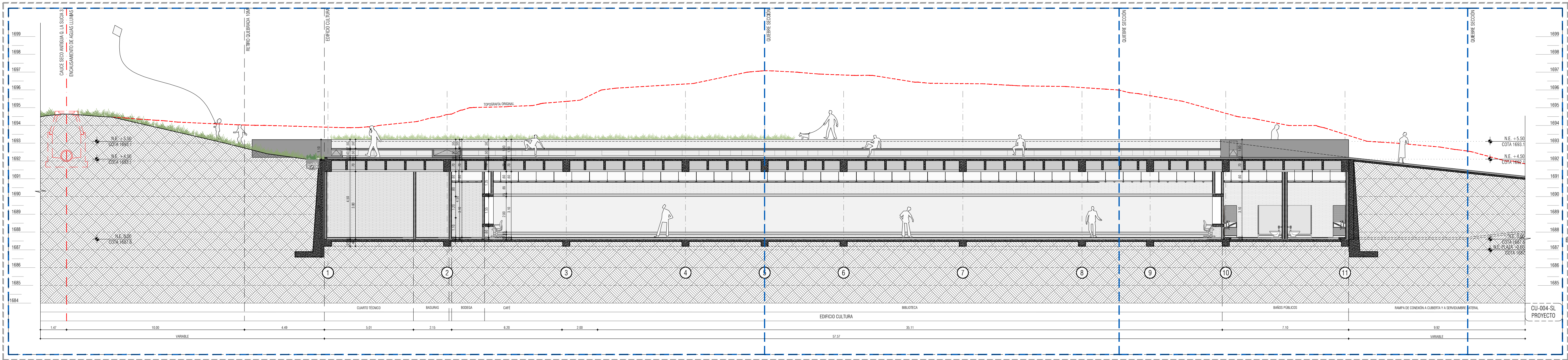
UPO-CU-004-SL/ Sección Longitudinal ESC 1:125
